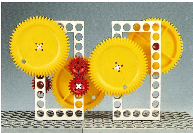
Engrenages - Fiche N° 5
