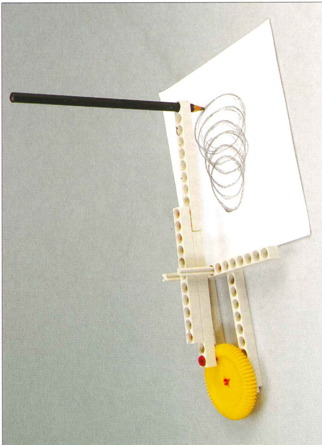
Machine à dessiner 1.
